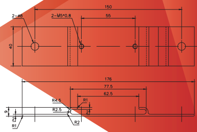
規格圖-吸頂
