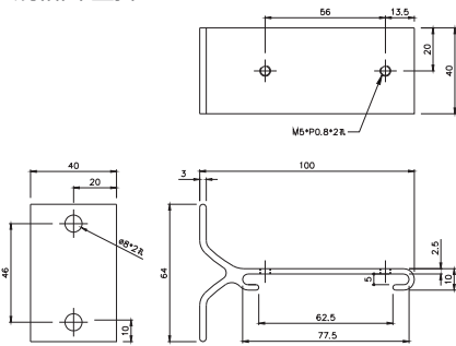
規格圖-壁掛
