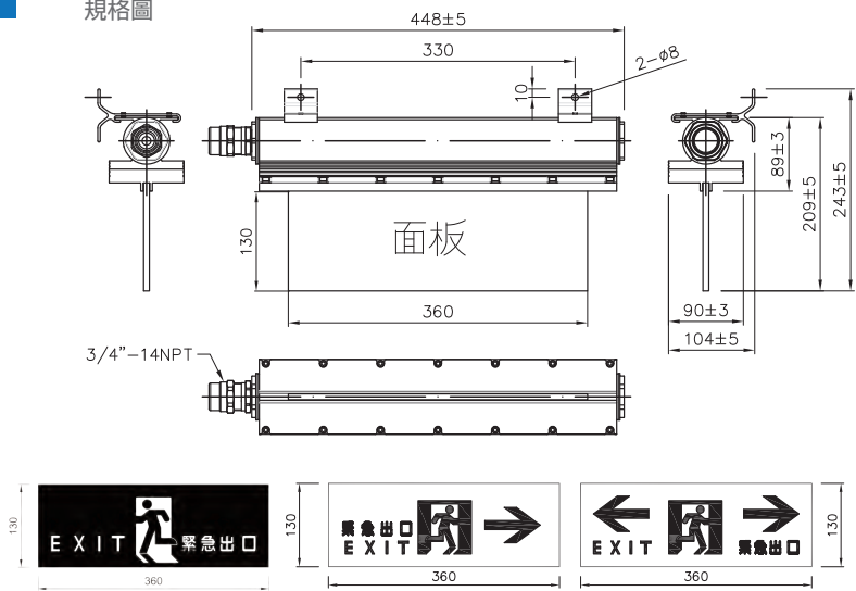
規格圖
