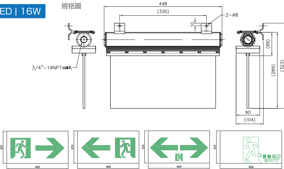
規格圖
