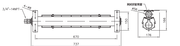
規格圖-19W
