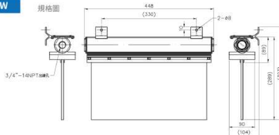
規格圖
