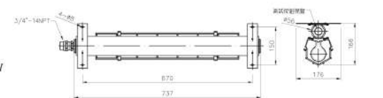
規格圖-19W
