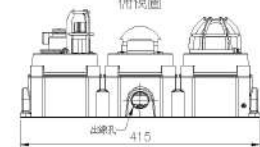
正視圖
