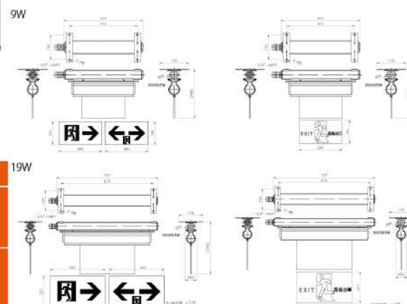
規格圖-吸頂
