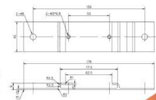
規格圖-吸頂
