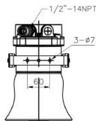
俯視圖
