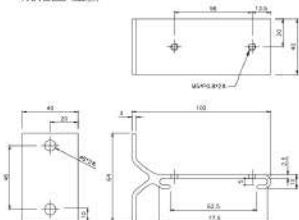
規格圖-壁掛
