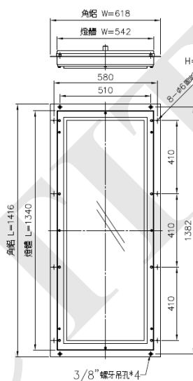
燈具尺寸-面掀
